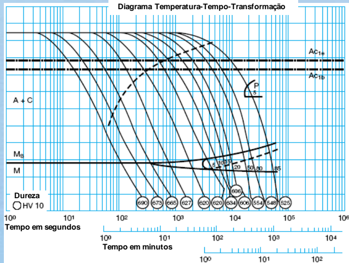
Diagrama Temperatura-Tempo-Transformação
